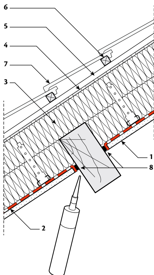
Figure 10.1 : Jonction rampant – panne apparente
