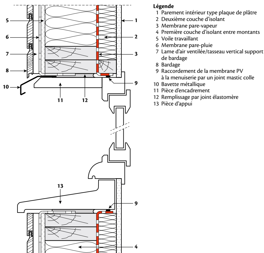
Figure 39.1 : Jonction mur – fenêtre ou porte
